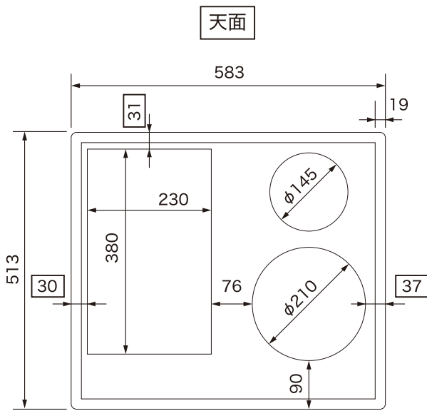
ワク内の数字はヒーターの外周から縁までの距離
